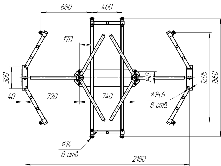
Установочные размеры турникета «Ростов-Дон ПР2/ЗМ2»
